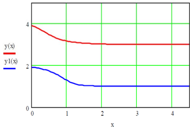
ნახ. 3. პროგრამა Mathcad-ზე და ტრაექტორია სხვადასხვა საწყისი:
